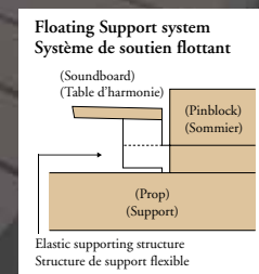
Upright piano soundboard structure Structure de la table d'harmonie d'un piano droit
